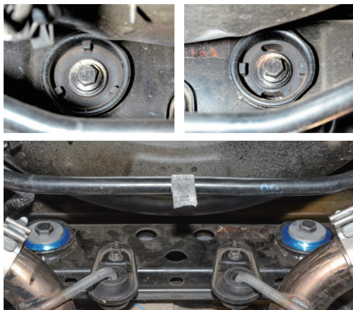
Illustration of installation-Rear 後方安裝示意圖
