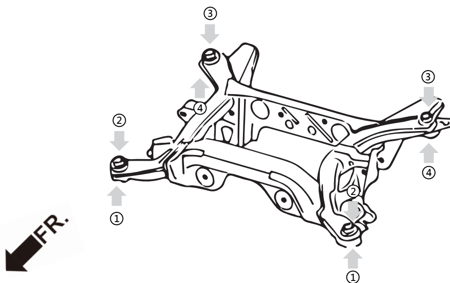
Illustration of installation-Front 前端安裝示意圖
